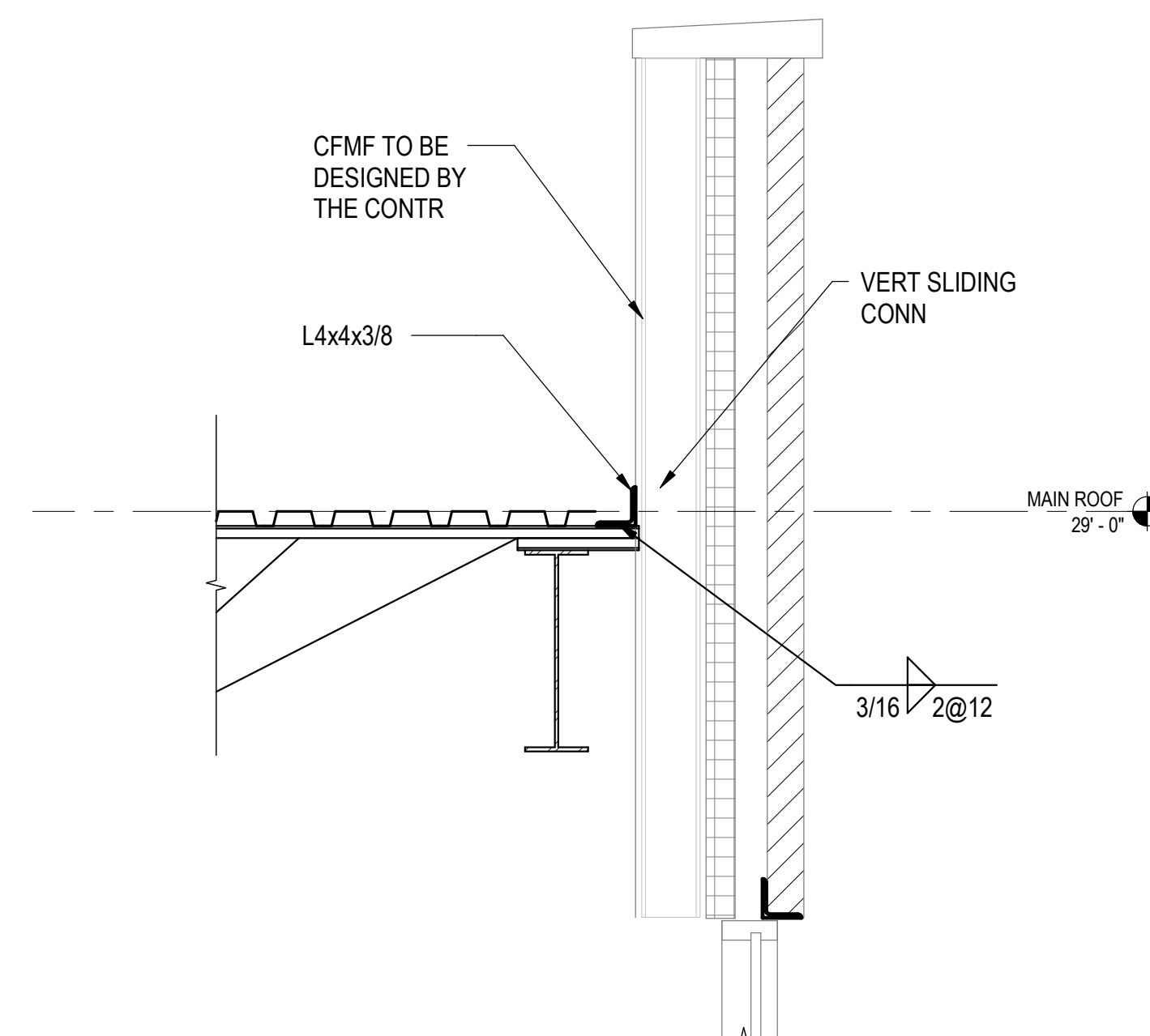
SECTION 8 SCALE: 3/4" = 1'-0" S-321
