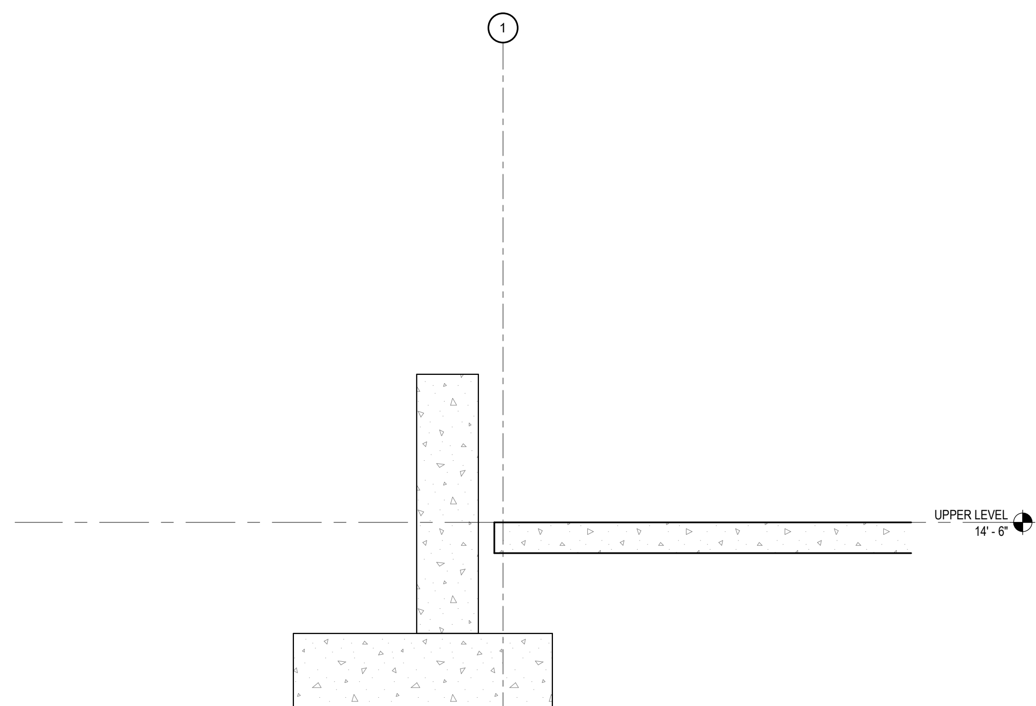
SECTION 8 SCALE: 3/4" = 1'-0" S-301
