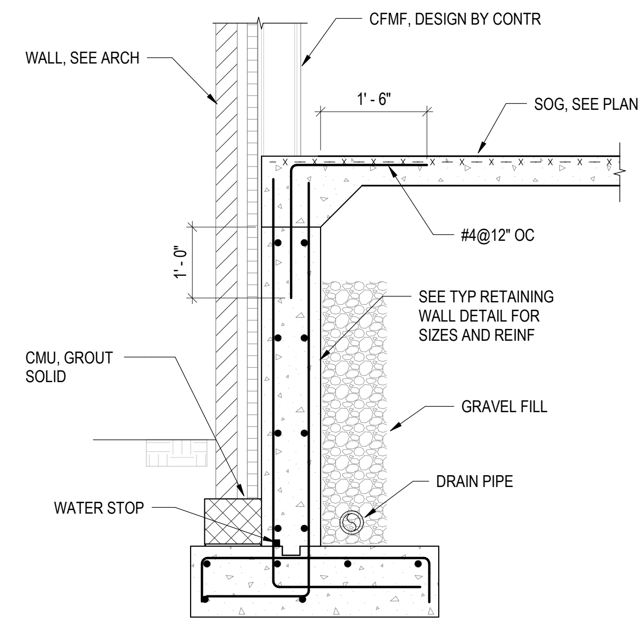
SECTION 4 SCALE: 3/4" = 1'-0" S-301
