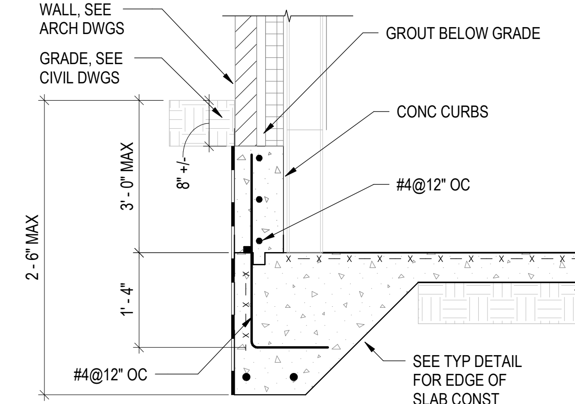
SECTION 4 SCALE: 3/4" = 1'-0" S-301
